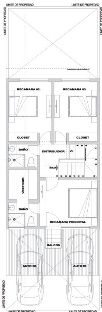
PLANTA ALTA
